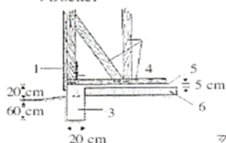
Verankerung von Gerüst und Sockel
