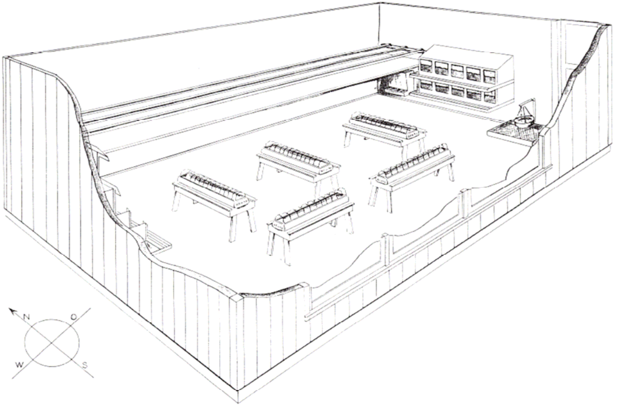
Vorbildliche Stalleinrichtung für 100 Hühner
