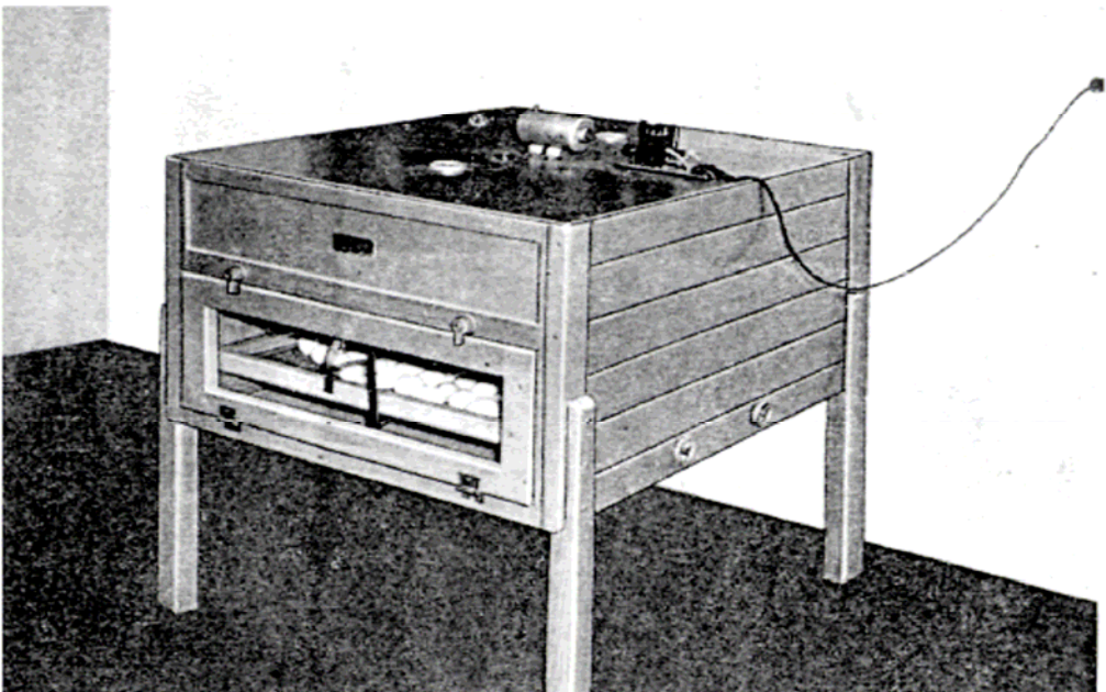
Flächenbrüter
