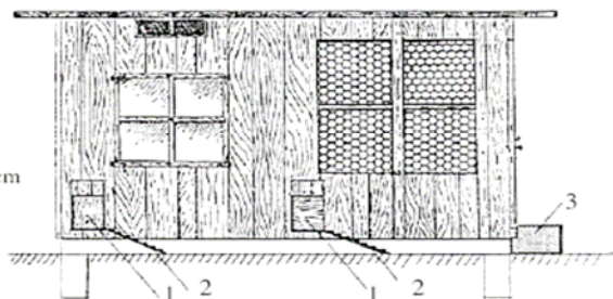
Vorderansicht eines Stalles
