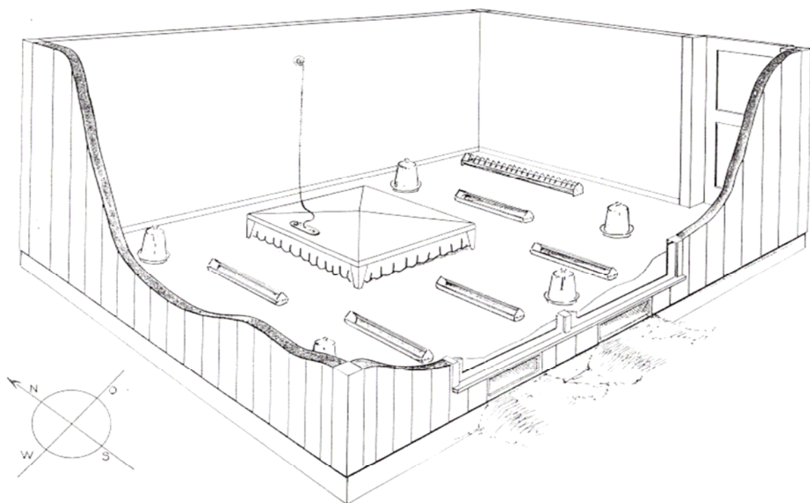
Vorbildliche Kükenstalleinrichtung mit Elektroglucke für 250 - 300 Küken
