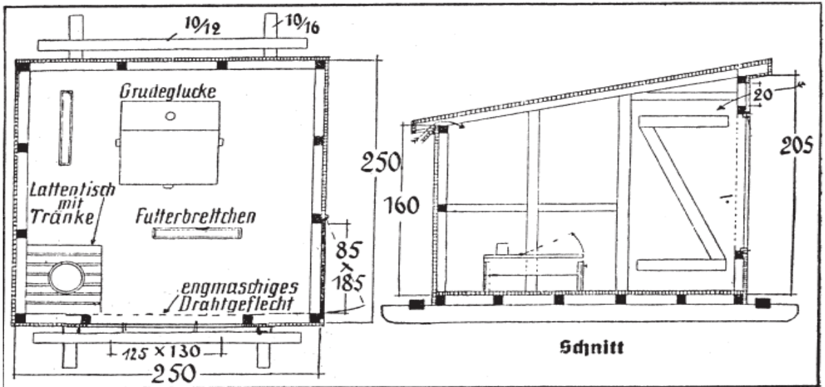
Grundriß und Querschnitt durch den Aufzuchtstall.
