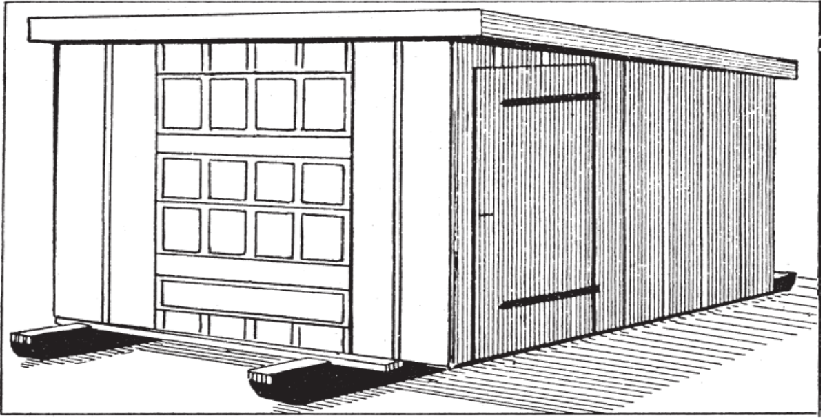
Aufzuchtstall auf Kufen für 200 - 250 Küken
