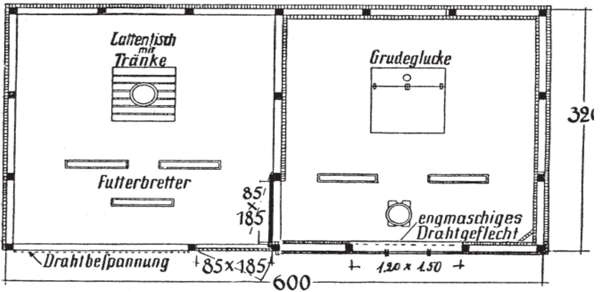
Grundriß zum Aufzuchtraum, mit Warm- und Kaltraum.
