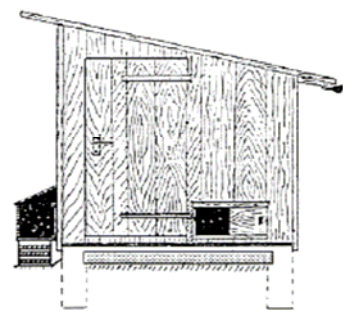
Stirnseitenansicht eines Hühnerstalles
